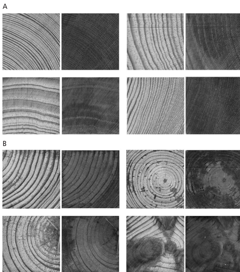
Fig. 1 : Echantillons de pin d'Alep après découpe dans le sens latéral avant et après application du réactif de chrome azurol S. (A) : Echantillons d'aubier. (B) : Echantillons de duramen.
